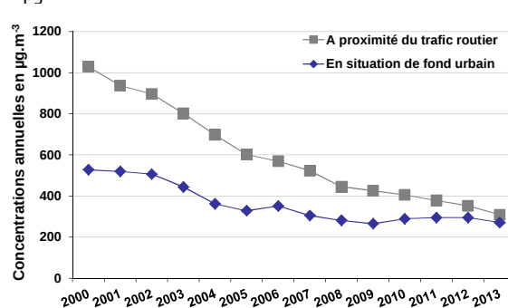
Figure D3.3-2 Évolution des concentrations annuelles de monoxyde de carbone (CO) dans l'air
