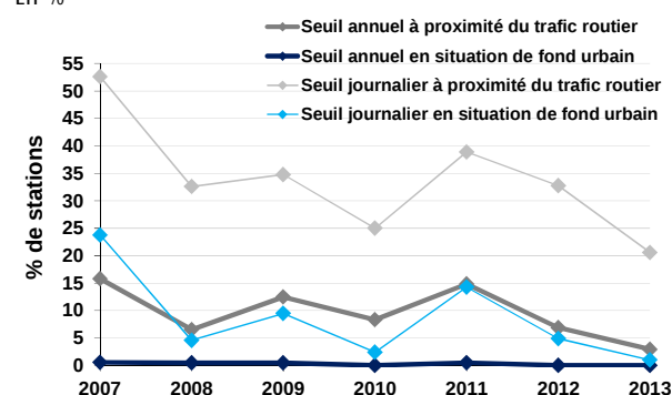
Figure D3.3-6 Évolution du pourcentage de stations de mesure qui ne respectent pas les seuils en particules \text{PM}_{10} pour la protection de la santé
