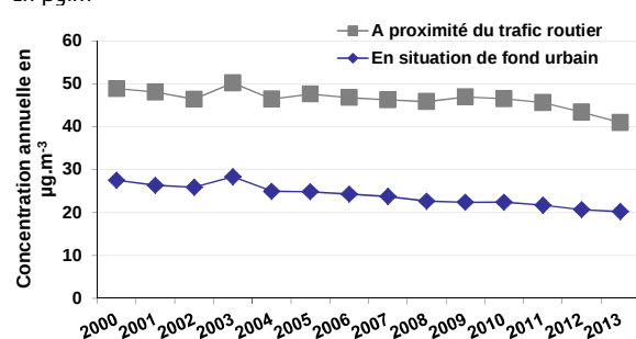
Figure D3.3-3 Évolution des concentrations annuelles de dioxyde d'azote ( \text{NO}_2 ) dans l'air
