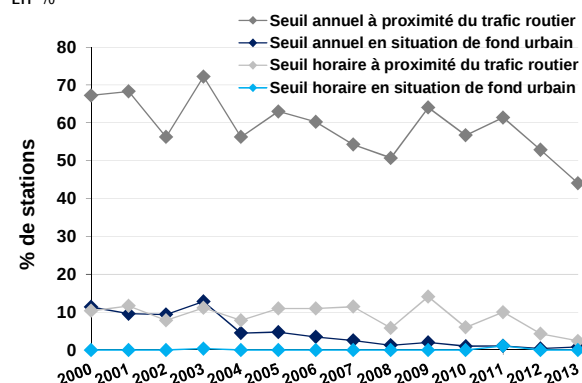
Figure D3.3-5 Évolution du pourcentage de stations de mesure qui ne respectent pas les seuils en dioxyde d'azote ( \text{NO}_2 ) pour la protection de la santé
